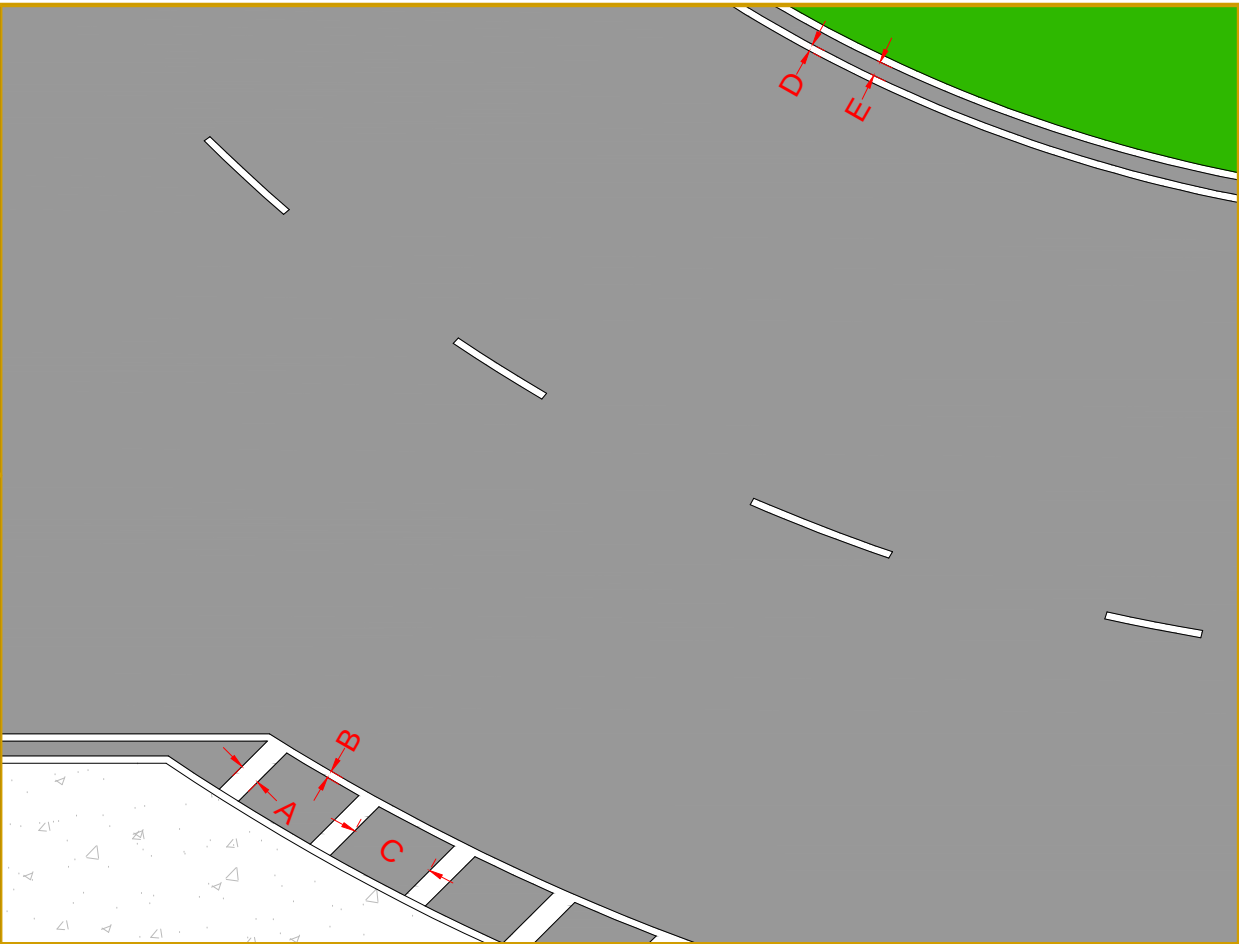
Zebrado de preenchimento da área de pavimento não utilizável Faixa de bordo rotatória
