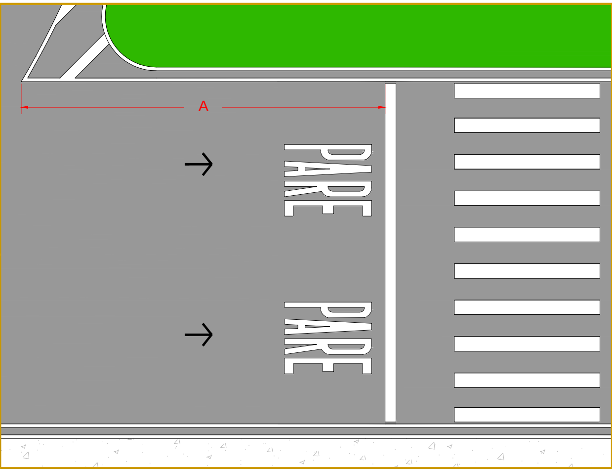
Recuo para parada de veículos antes da faixa de pedestre
